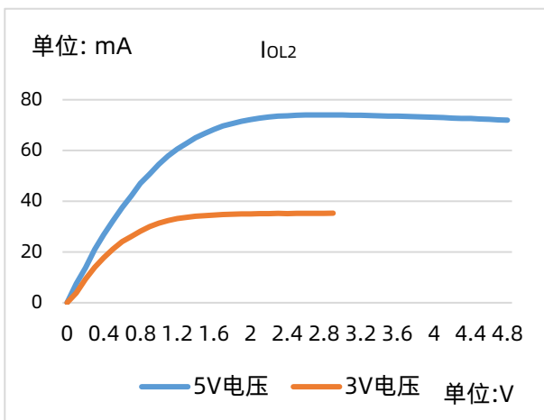
普通驱动模式下灌电流
